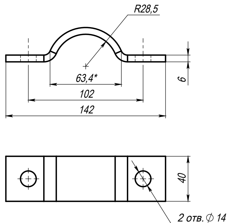
Поз.1 (Полухомут)
