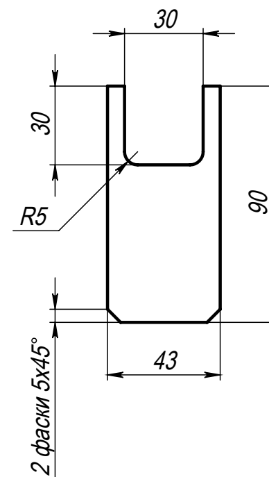
Поз.4 (Ребро внутреннее)
